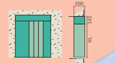
Façade complète avec linteau réduit (2)
