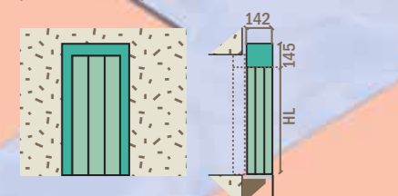
Porte en éléments séparés pour cadre de porte battante conservé (4)
